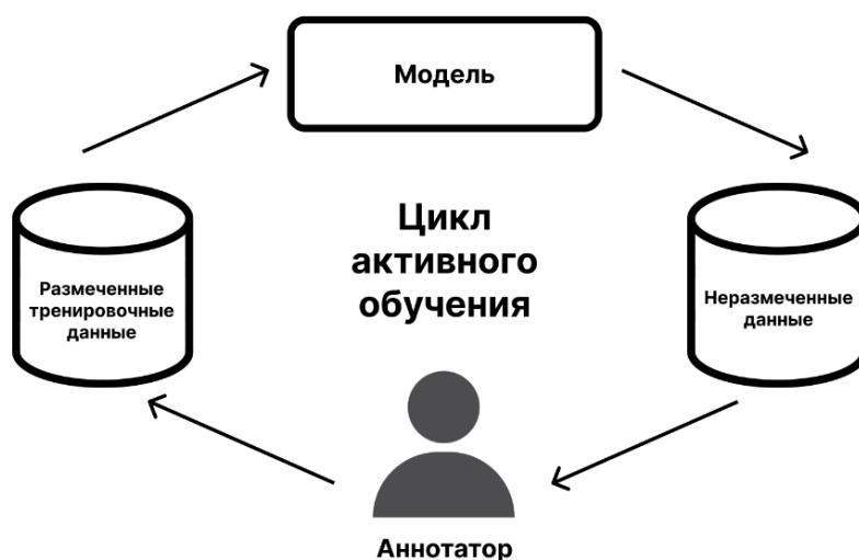
Рисунок 1 – Схема процесса активного обучения
